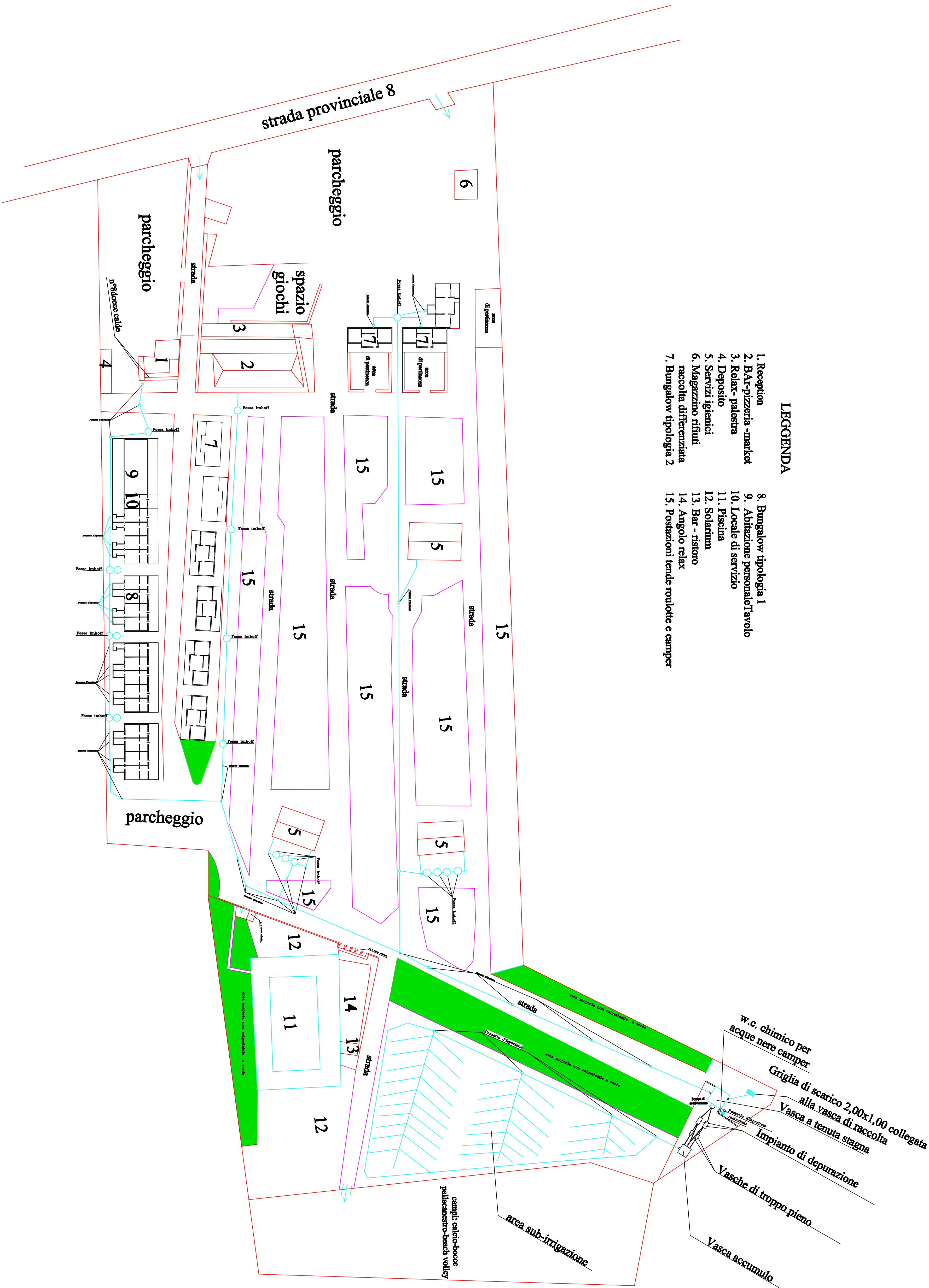
PLANIMETRIA GENERALE SCALA 1:500
