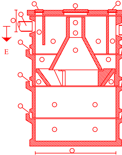
SEZIONE A-B
