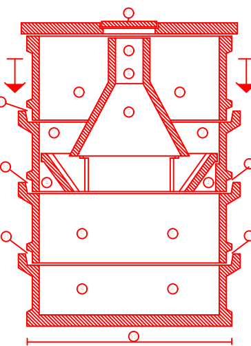
SEZIONE C-D
