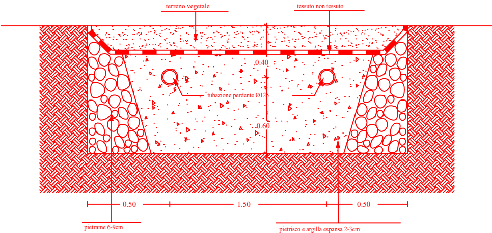
SEZIONE CONDOTTA SUBIRRIGANTE
