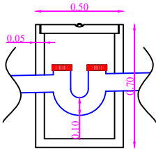
PART. POZZETTO SIFONATO SCALA 1:20
