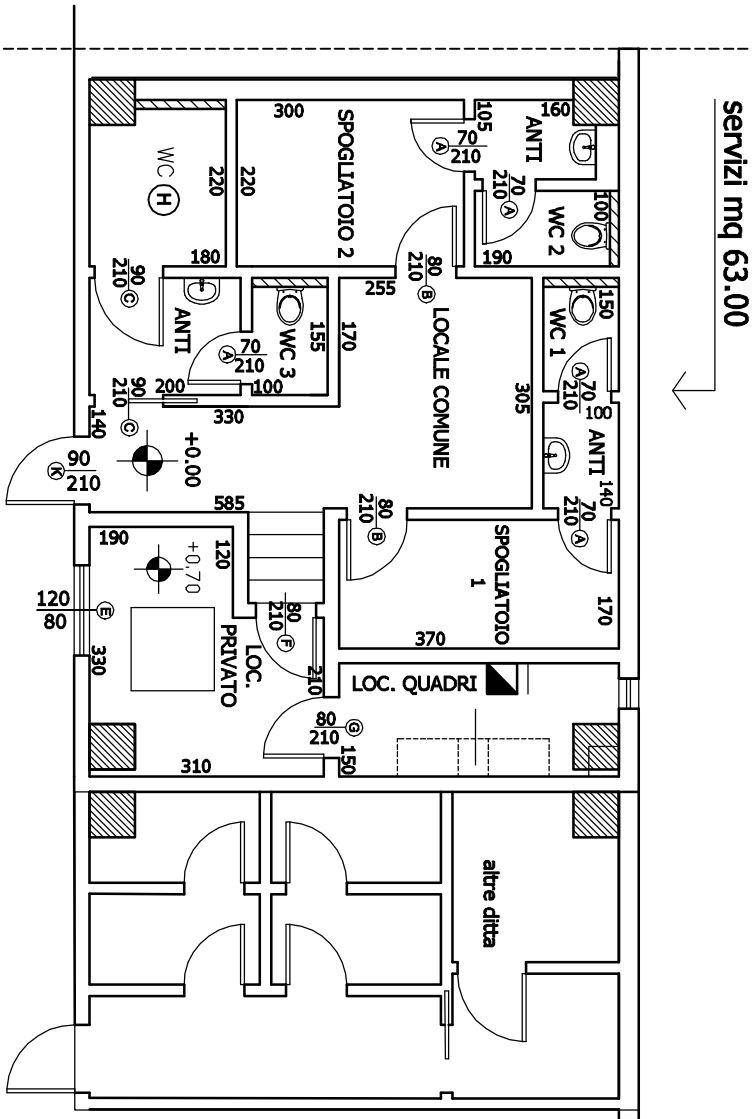
PARTICOLARE ZONA SERVIZI IGIENICI
