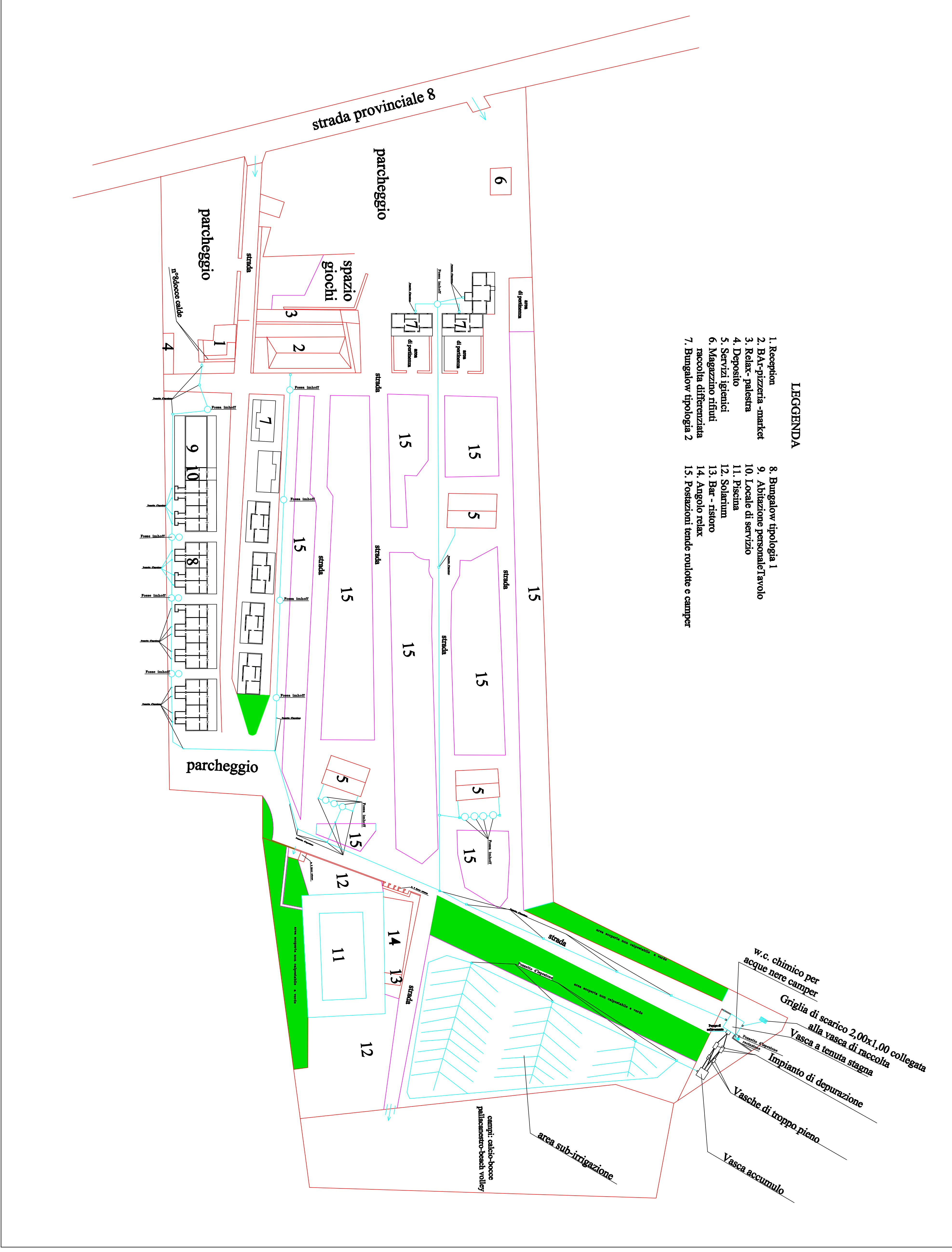
PLANIMETRIA GENERALE SCALA 1:500
