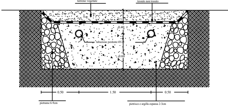
SEZIONE CONDOTTA SUBIRRIGANTE
