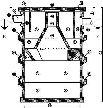
SEZIONE A-B
