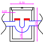
PART. POZZETTO SIFONATO SCALA 1:20
