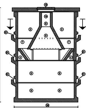
SEZIONE C-D
