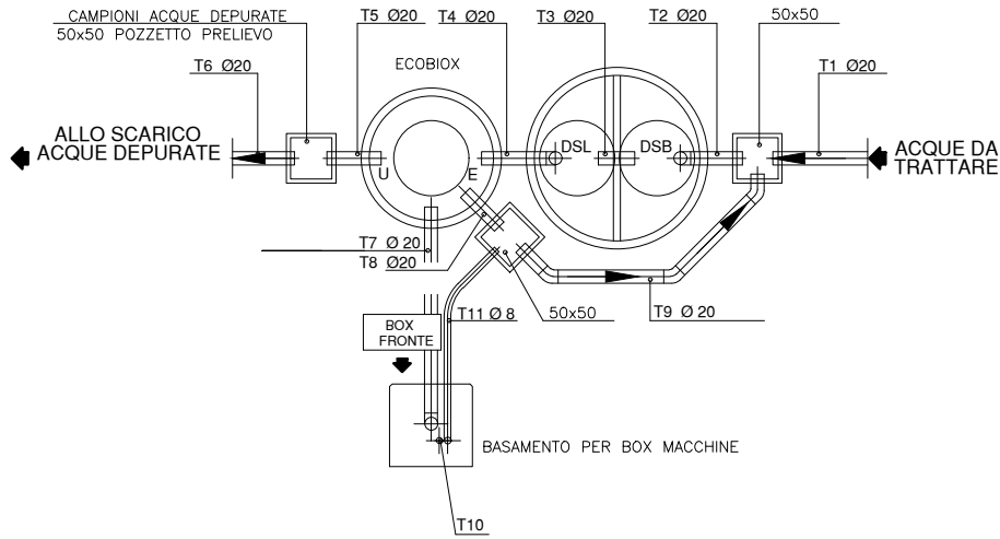
schema di processo depurativo delle acque di lavaggio
